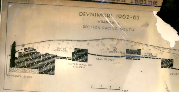
23. Vihara II : Section facing
